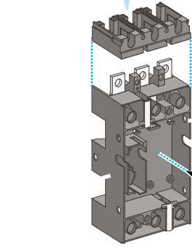
Mühürlenabilir terminal koruyucuları
